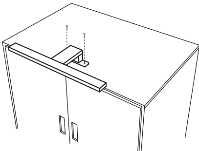
Монтаж върху шкаф
