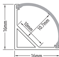
Алуминиев профил, черен, с черен дифузер и черни тапи в комплекта
