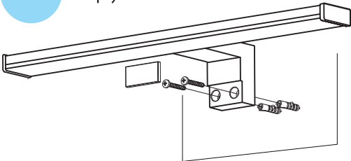
Монтаж върху стена
