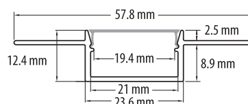
Алуминиев профил за гипсокартон, с черен дифузер и черни тапи в комплекта
