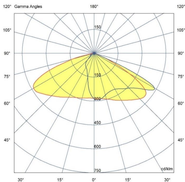
СВЕТЛОРАЗПРЕДЕЛИТЕЛНА ДИАГРАМА
