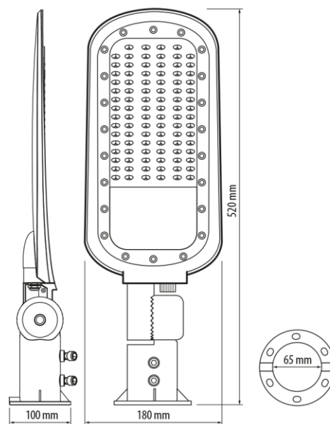
РАЗМЕРИ
