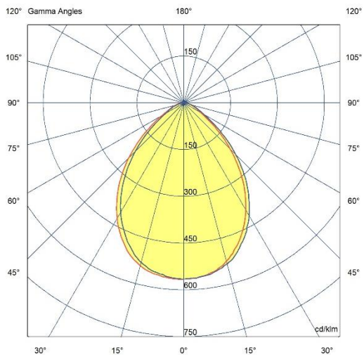
СВЕТЛОРАЗПРЕДЕЛИТЕЛНА ДИАГРАМА
