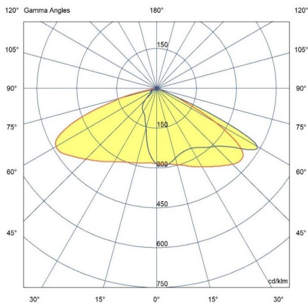
СВЕТЛОРАЗПРЕДЕЛИТЕЛНА ДИАГРАМА
