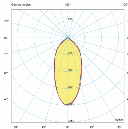
СВЕТЛОРАЗПРЕДЕЛИТЕЛНА ДИАГРАМА С ДИФУЗЕР 45° (LSFL45)
