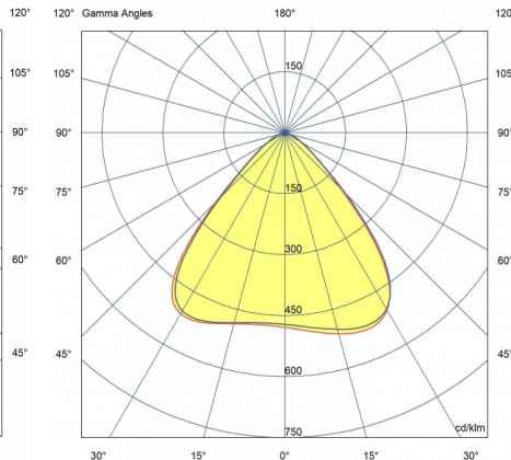
СВЕТОРАПРЕДЕЛИТЕЛНА ДИАГРАМА С ДИФУЗЕР 90°
