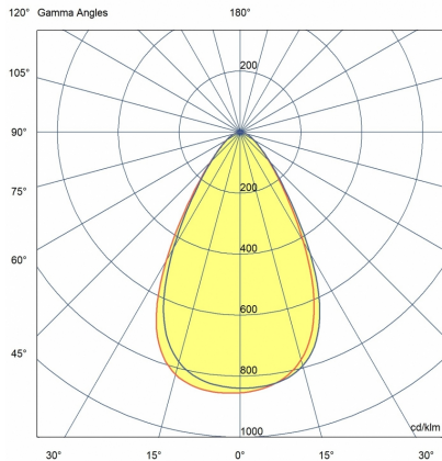
СВЕТОРАПРЕДЕЛИТЕЛНА ДИАГРАМА С ДИФУЗЕР 60°
