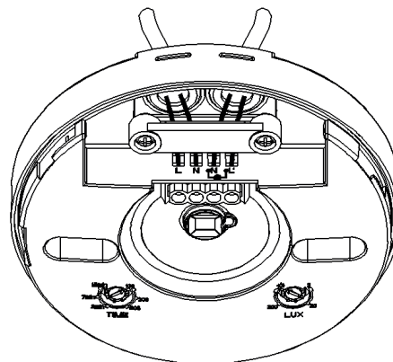
Окабеляване през отворите на основата
