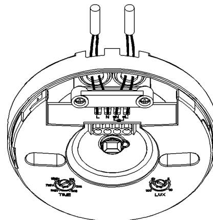
Окабеляване през страничните отвори
