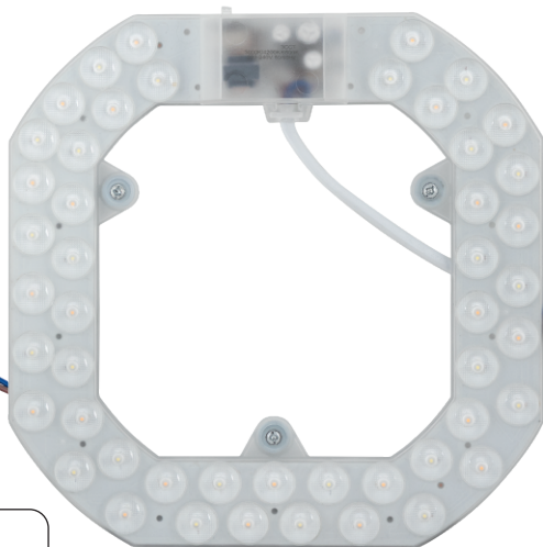
LMM24CCT 193×193×23 mm
